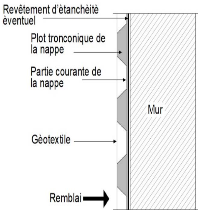
Figure 2 - Sens de pose des nappes T KONE G DRAIN
