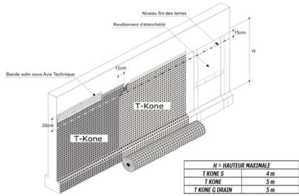
Figure 6b Pose sur étanchéité si la hauteur à traiter est supérieure à la largeur des lés
