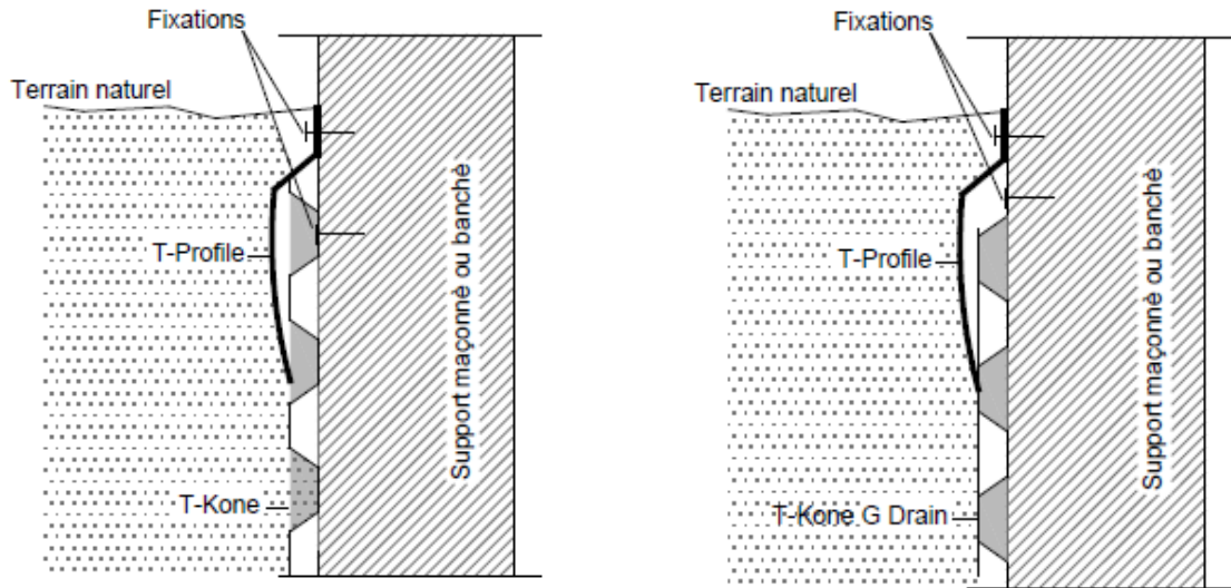
Figure 3 bis - Moulure T PROFIL PEHD
