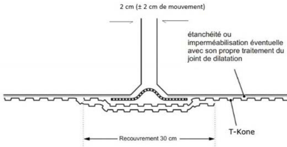
Figure 8 - Traitement des joints de dilatation - Zones de sismicité (arrêté du 22 octobre 2010 modifié) conduisant à des ouvertures de joints inférieures ou égales à 2 cm
