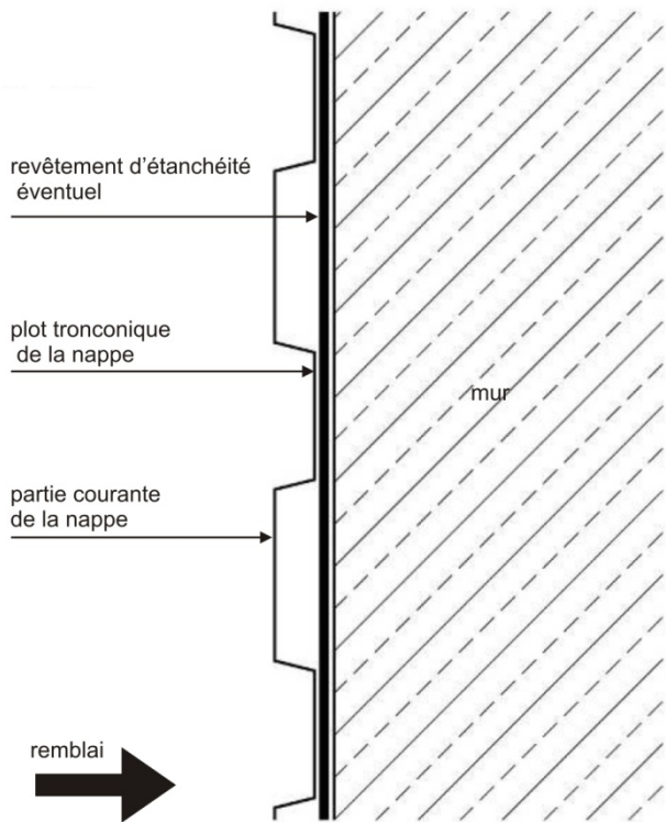
Figure 1 - Sens de pose des nappes T KONE S et T KONE
