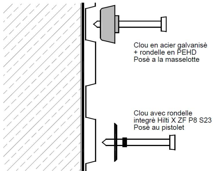
Figure 4 - Fixation haute des nappes T KONE S et T KONE sur support en maçonnerie
