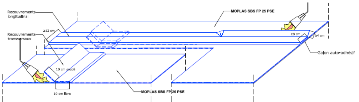
Figures 3 – MOPLAS SBS FP 25 PSE Recouvrements à double galon
