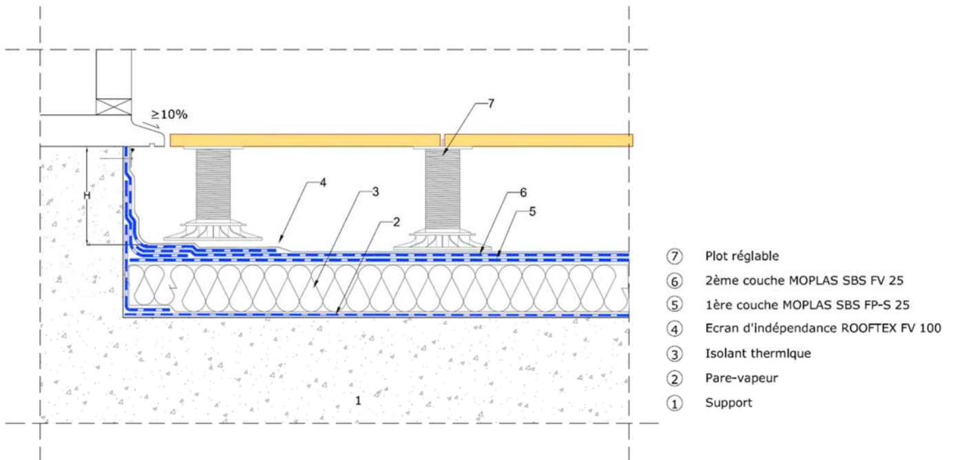
Figures 2b – Relevés et protection des relevés (principe)
