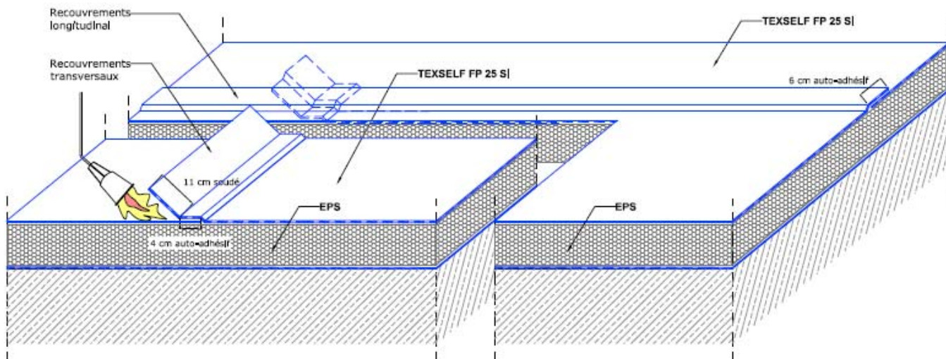
Figure 4 – TEXSELF FP 25 SI Recouvrements à double galon (uniquement sous protection rapportée)
