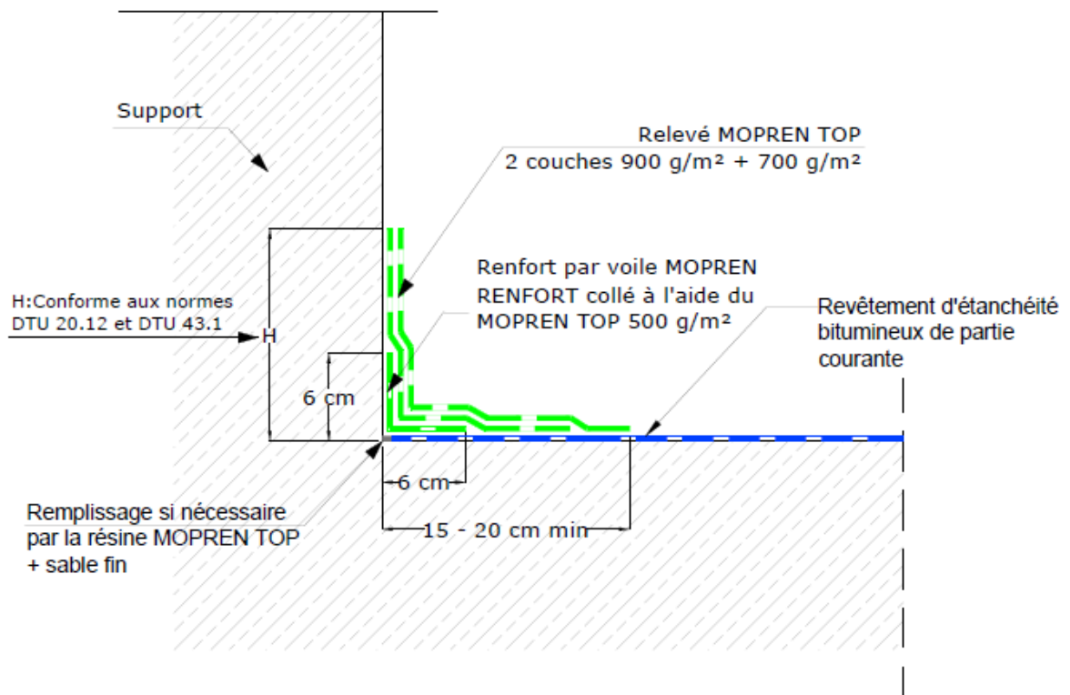
FIGURE 6b – Mise en œuvre du procédé MOPREN TOP - Cas particulier sans dispositif écartant les eaux de ruissellement
