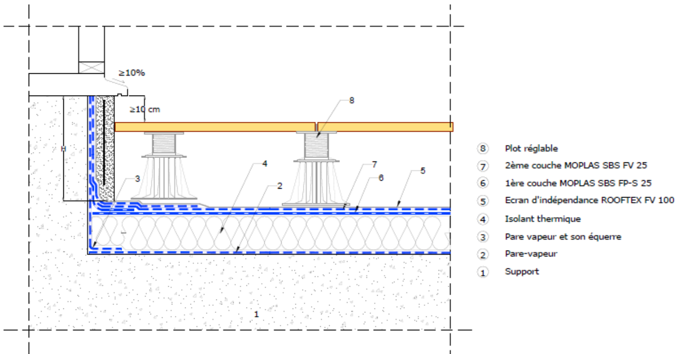
Figures 2a – Seuils à relief
