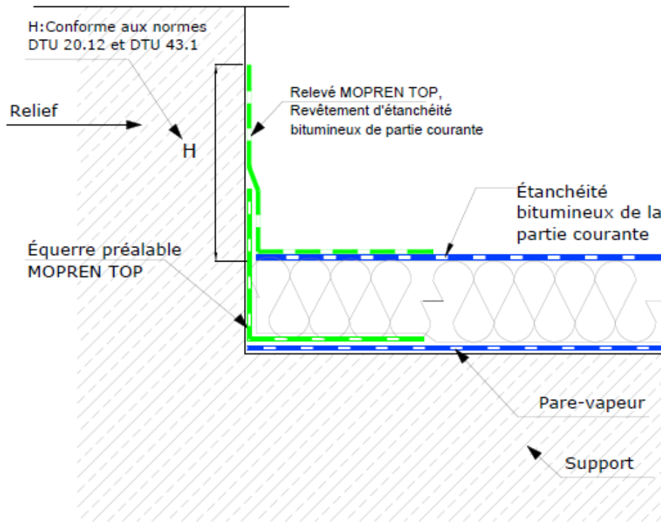
Figure 6a - Procédé MOPREN TOP Principe - Cas particulier sans dispositif écartant les eaux de ruissellement
