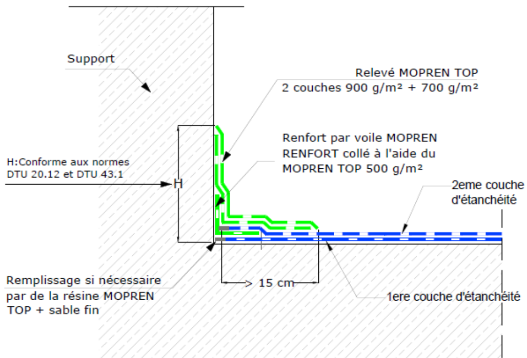
FIGURE 6c - Procédé MOPREN TOP - variante de pose de l'équerre de renfort insérée entre les deux feuilles du revêtement bicouche - Cas particulier sans dispositif écartant les eaux de ruissellement
